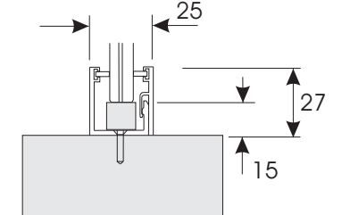
Section D-D
